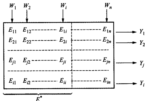
既然发动机的输入的个数大于输出的个数,所以,如果希望完全确定系统的运转状态,除了要设法使所有输出 Y_v(s) 随预定的数值 X_j(s) ( j=1,2,\dots,i ) 相应地变化之外,还要设法使变数 W_\mu(s) ( \mu=i+1,i+2,\dots,n ) 也取预定的数值 \Xi_\mu(s) 。因此,被控制量就是 i 个输出 Y_v(s) ( v=1,2,\dots,i ) 和 n-i 个发动机输入 W_\mu(s) ( \mu=i+1,i+2,\dots,n )。如果由测量仪器对 W_\mu(s) 所测出来的值是 \gamma_\mu(s) ,那么,误差就是 \Xi_\mu(s) - \gamma_\mu(s) 。发动机的输出的偏差的定义是 X_v(s) - Z_v(s) , Z_v(s) ( v=1,2,\dots,i ) 就是 Y_v(s) 经过测量仪器所测量出的数值,就像图 5.1 的那种情形。控制的作用就在于把这些偏差当作输入来产生伺服马达的改正信号 U_k(s) 。这就是系统的反馈作用。在我们所讨论的一般的系统(5.4)里,改正信号 U_k(s) 与所有偏差的关系是线性的。既然有 n 个偏差信号,也就有 n 个改正信号,所以 k=1,2,\dots,n 。因此就有
